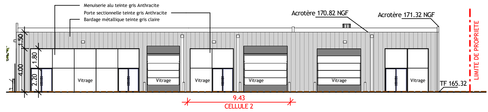
Façade Sud
