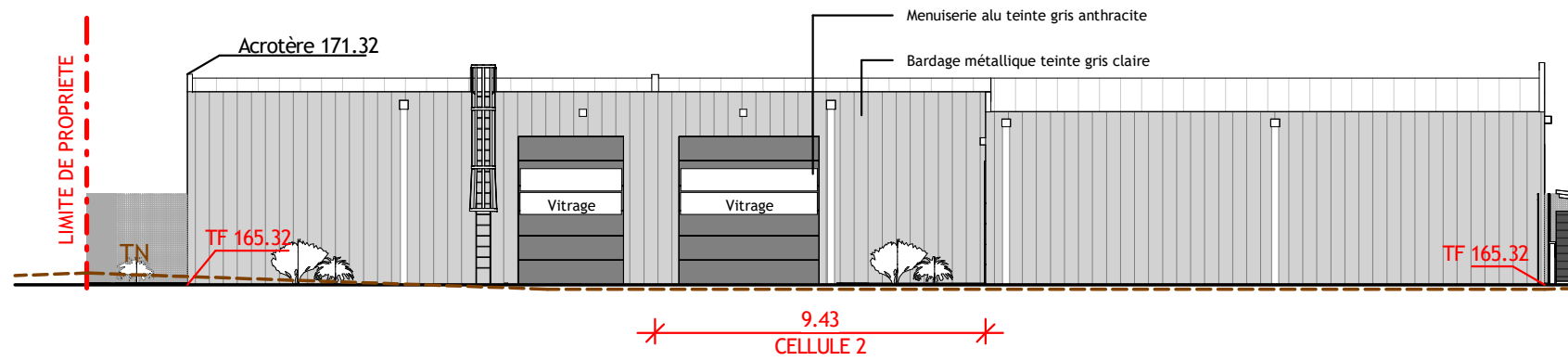
Façade Nord
