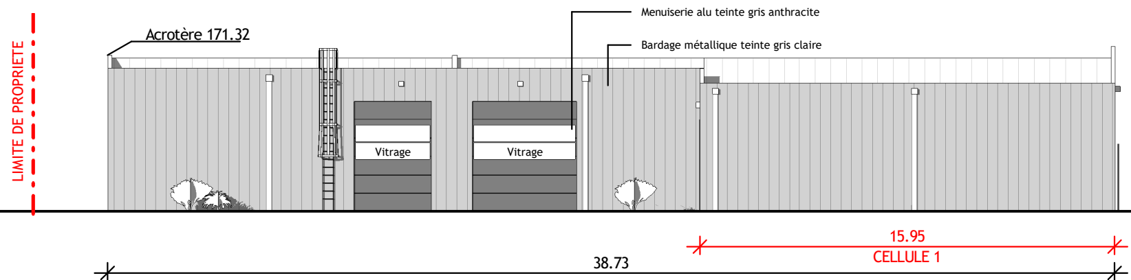
Façade Nord
